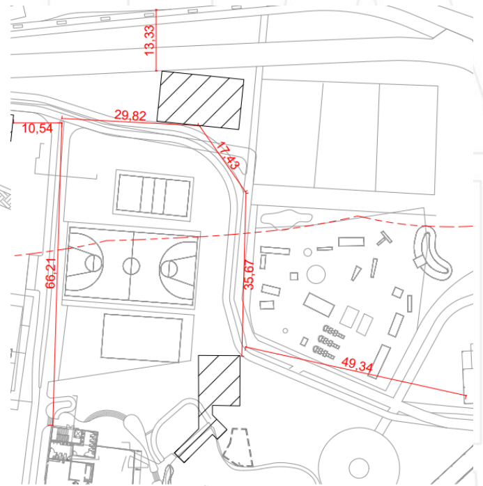
PLANTA BAIXA | IMPLANTAÇÃO ESCALA 1:500
